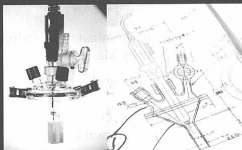
写真は特注品の参考例と、特注品の図面です
